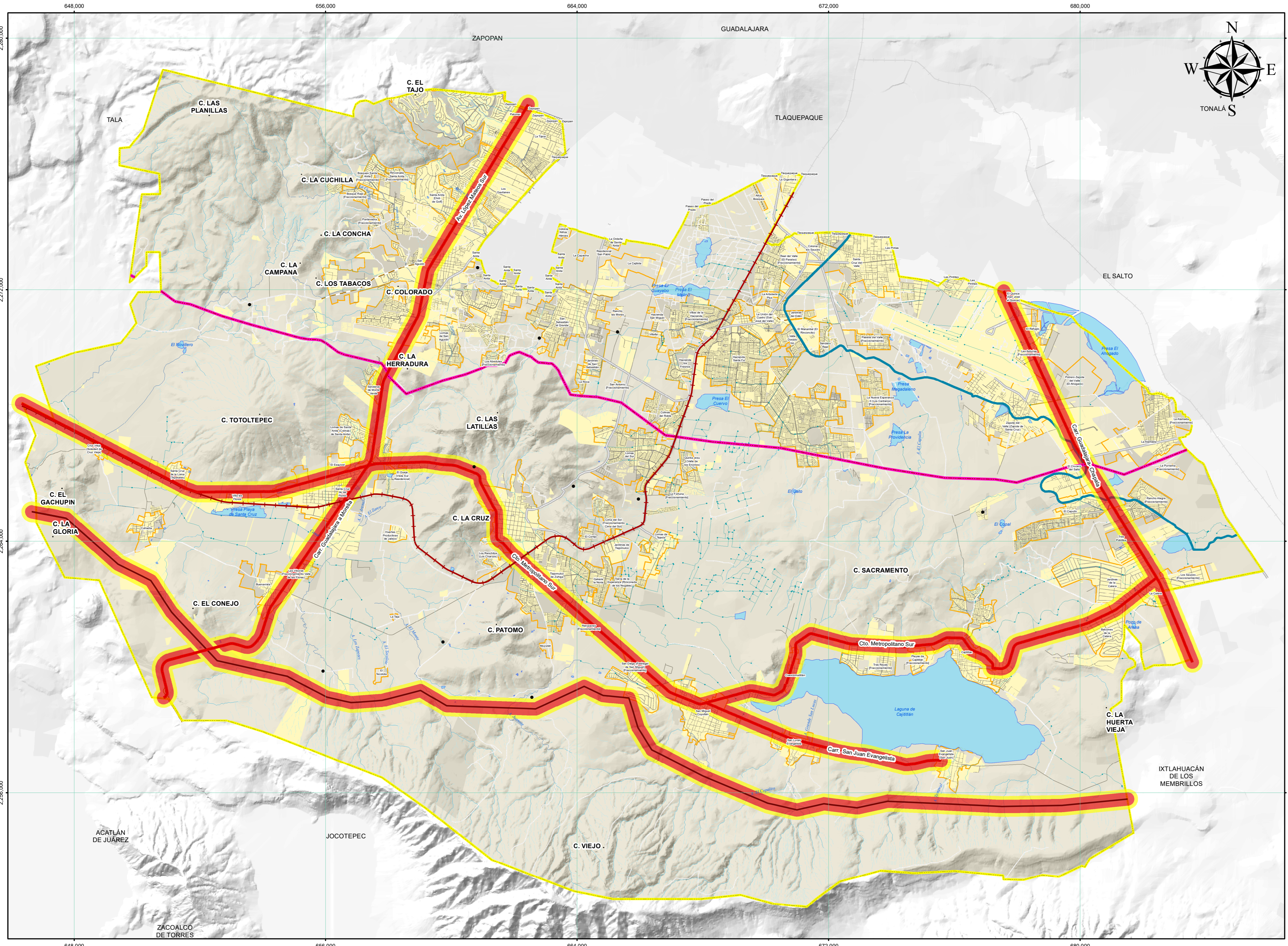
Mapa 4.24 Simulación del nivel de peligrosidad por transporte de sustancias peligrosas en carretera Distancia de afectación por nube tóxica por acetileno 78kg
